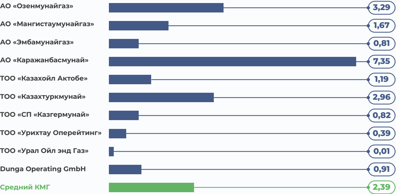
УДЕЛЬНОЕ ПОТРЕБЛЕНИЕ ЭНЕРГИИ НА ДОБЫЧУ 1 Т УВС, ГДЖ/Т
